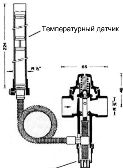
Сильфонная система
